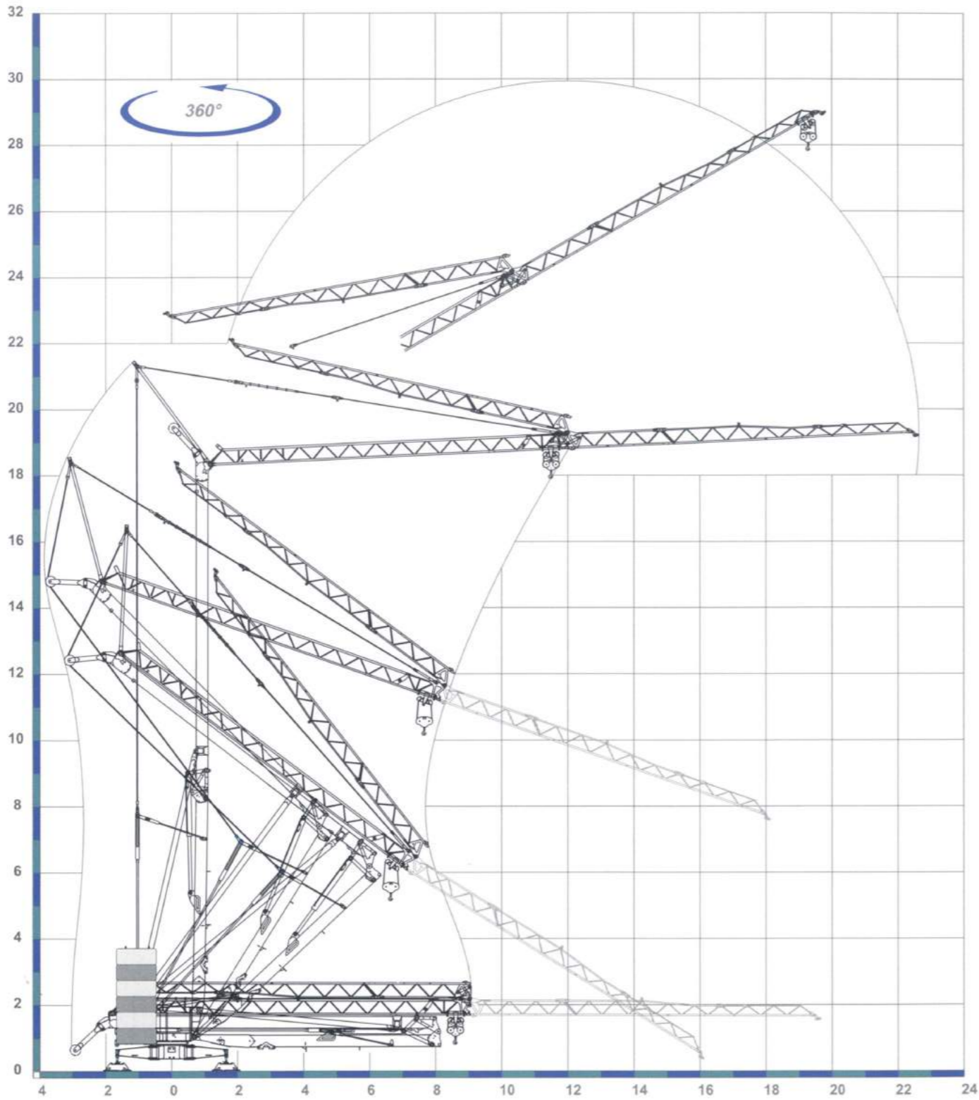
Sequenza di montaggio su 360°. Aufstellvorgang uber 360°. Déroulement de montage sur 360°. Erection procedure on 360°. Montaje sobre 360°.
